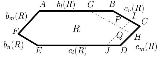
Fig. A-6. For Lemma 7
