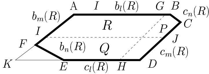
Fig. A-3. For Lemma 4
