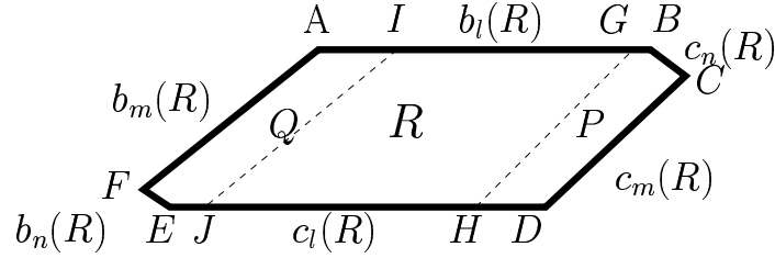
Fig. A-4. For Lemma 5.
