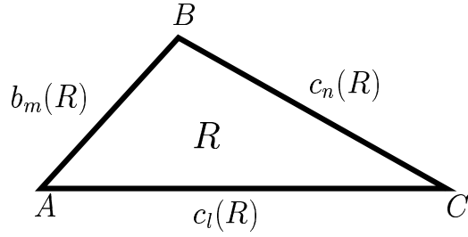
Fig. A-1. For Lemma 2
