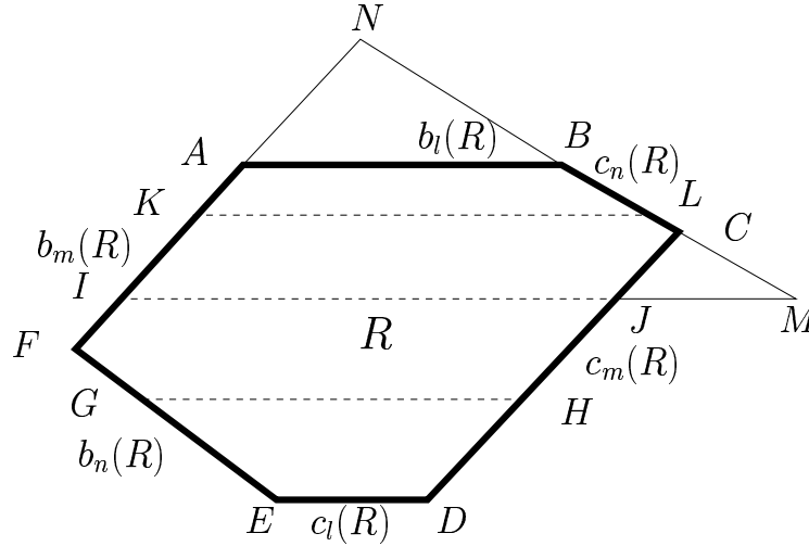
Fig. A-2. For Lemma 3
