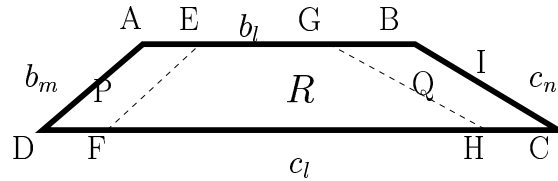
Fig. A-5. For Lemma 6
