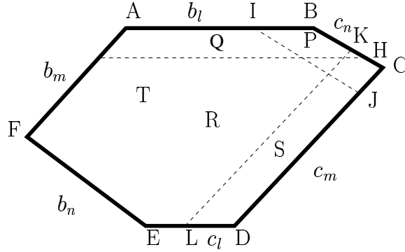
Fig. A-7. For Lemma 8
